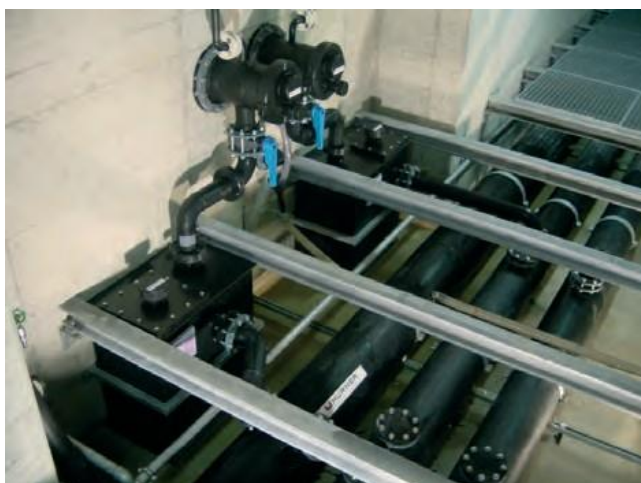
Deponieentwässerung mit Kontrollschacht und Bypass-Leitungen aus PE HD, ergänzt mit PE-EL Abluftleitung
