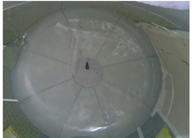
Klöppelboden eines Tankwagens in Arbeit
