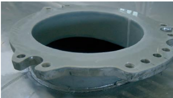
Chemikalienbeständige Verkleidung von Anschlussstutzen
